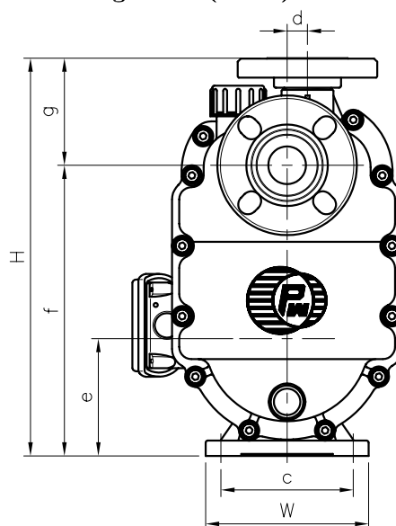
NH-PW-N Dimensions in mm
